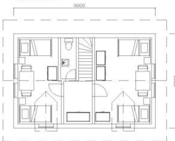
PUDORYS PODKROVÍ
