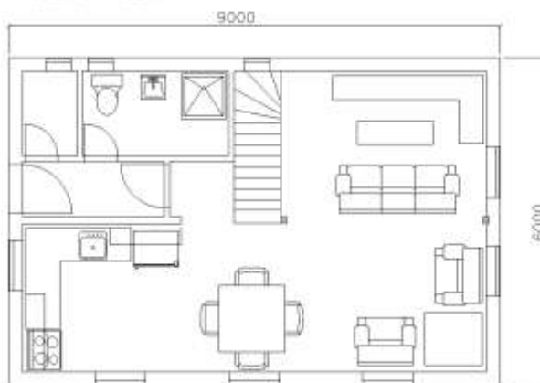
PUDORYS PRÍZEM'
